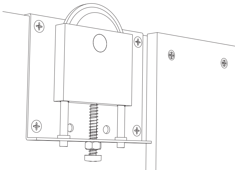
а. установка роликов на фасады
